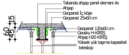
Şek.1 Sistemin enine kesiti
