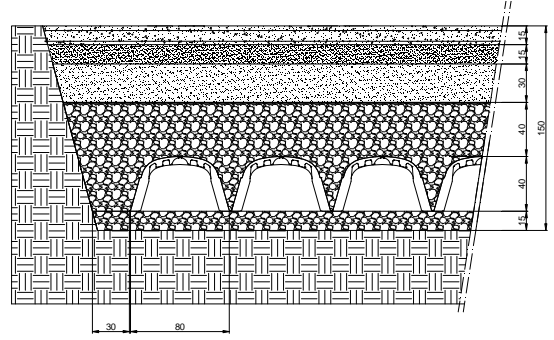
Şek.1 – Sistemin enine kesiti
