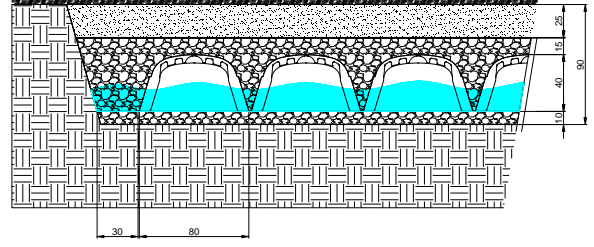
Şek. 1 – Sistemin enine kesiti
